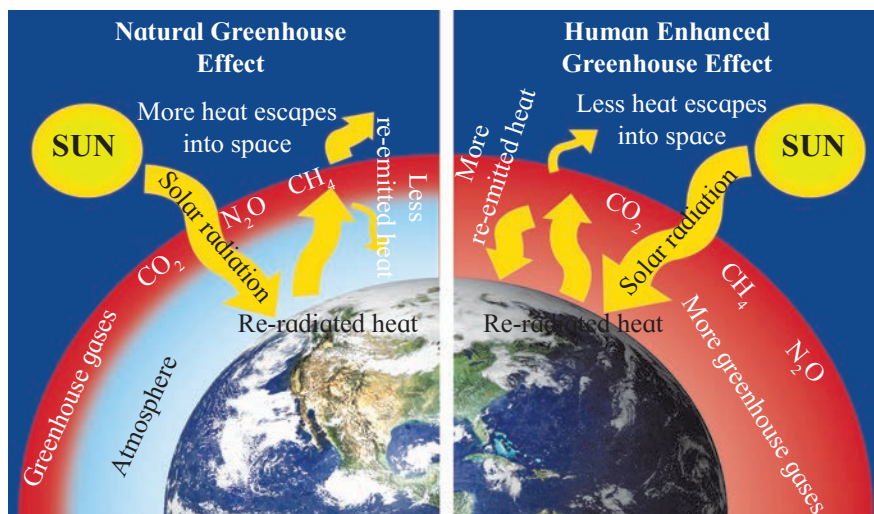
Fig. 15.10 : Greenhouse effect
