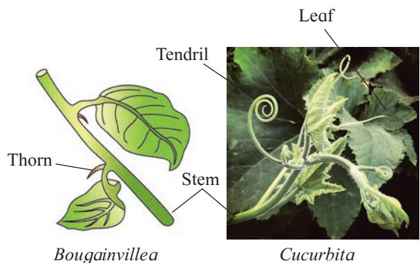
Fig. 5.12 : Homologous organs
