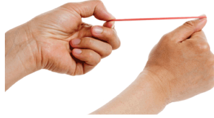
१३.३: ताणलेला रबरबँड
