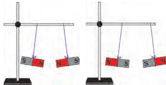
१५.१० : प्रेरित चुंबकत्व
