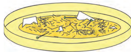
१५.२ : चुंबक
