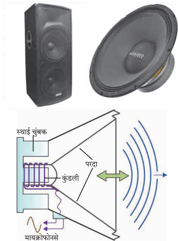
15.6 ध्वनिक्षेपक की अंतरिक रचना
