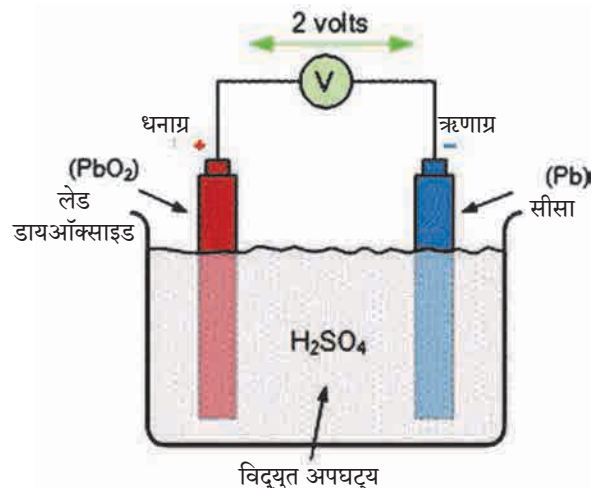
4.3 लेड-अम्ल विद्युतसेल
