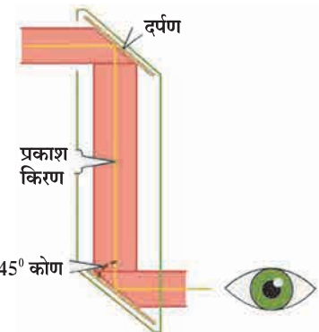
16.6 परिदर्शी
