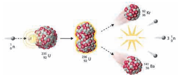
5.11 यूरेनियम - 235 का विखंडन
