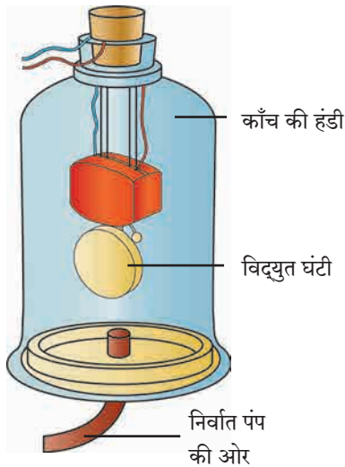
15.3 : ध्वनी संचलन के लिए माध्यम की आवश्यकता होती है।
