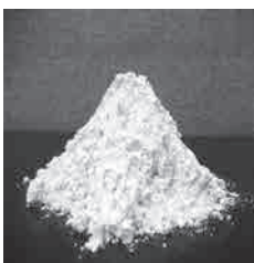
कैल्शियम हाइड्रॉक्साइड Ca(OH)_2
