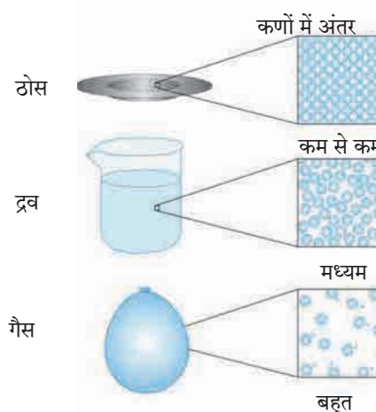
6.2 द्रव्य की भौतिक अवस्थाएँ : अतिसूक्ष्म स्तर पर चित्र
