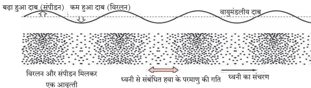
15.4 : ध्वनि तरंगों में विरलन और संपीडन इनकी आवृत्ति व हवा के दाब में परिवर्तन
