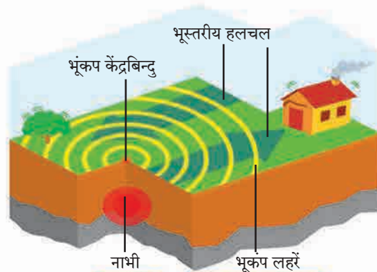
9.2 : भूकंपनाभि और भूकंपकेंद्र
