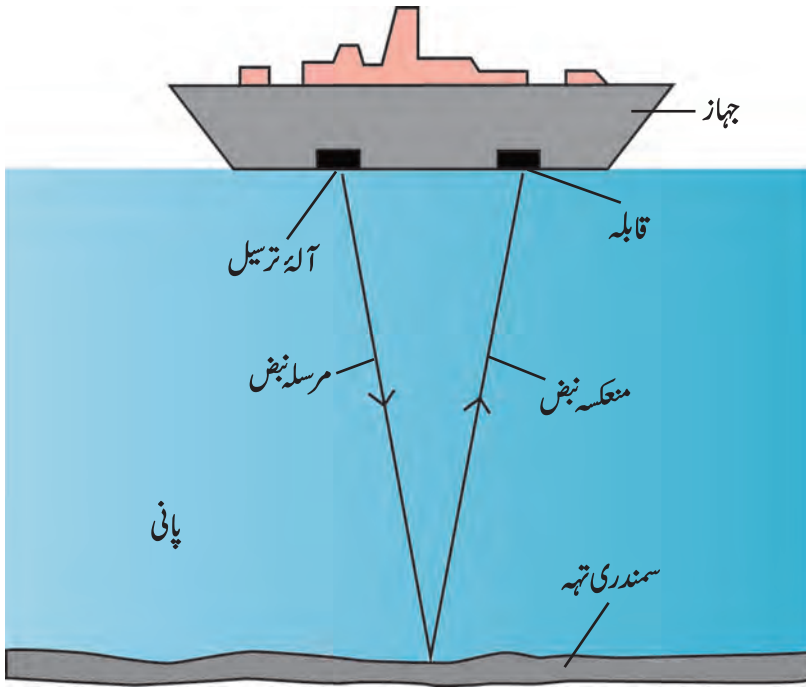
12.4: سونار سسٹم
