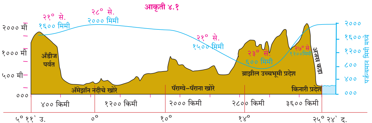
आकृती ४.२ : ब्राझीलच्या प्राकृतिक रचनेची छेद रेखा
