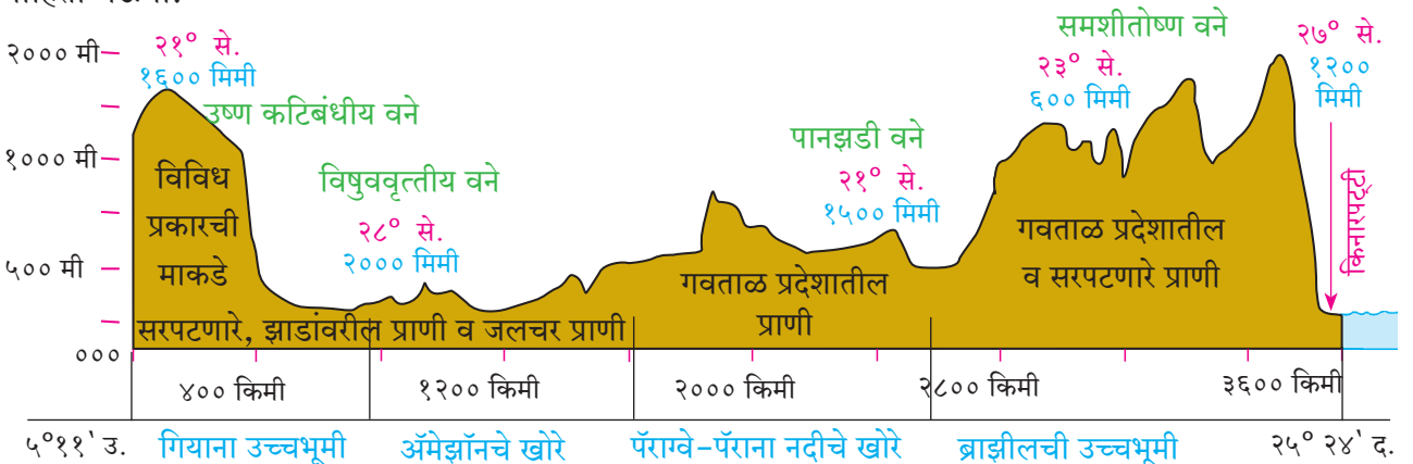
आकृती ५.२ : भूचरना, प्रमुख वनस्पती व प्राणी
