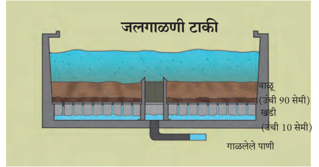
जलगाळणी टाकी
