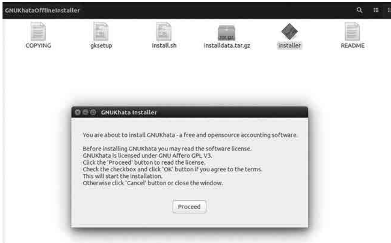
Fig. 1 : GNUKhata Installer
