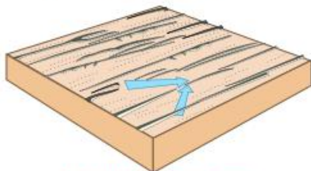
Fig. 3.26 : Linear or Seif dunes
