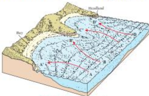
Fig. 3.8 : Wave refraction
