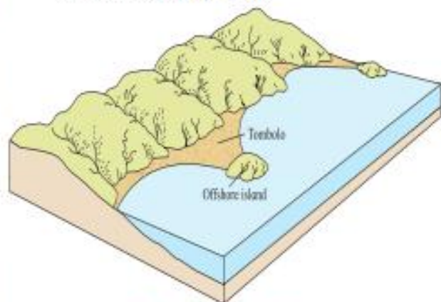
Fig. 3.14 : Tombolo
