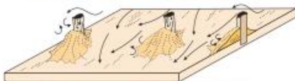
Fig. 3.22 : Formation of sand dunes
