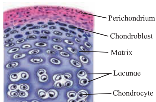
Fig. 10.12 Hyaline Cartilage
