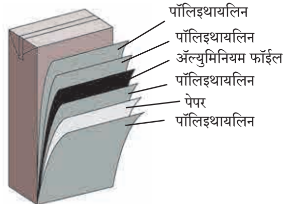
आकृती 14.20 : टेट्रा ब्रीक असेप्टिक पॅकेजिंग
