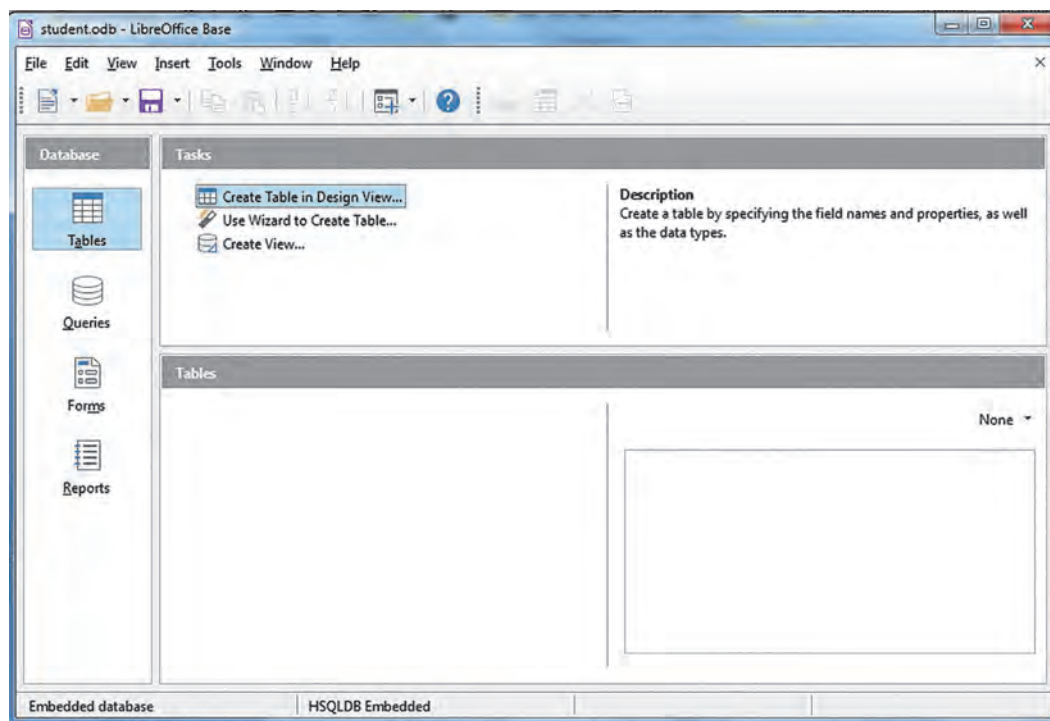
Fig. 5.1 : Database
