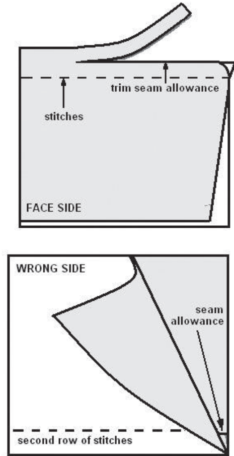
आकृती ४.१ फ्रेंच शिवण
