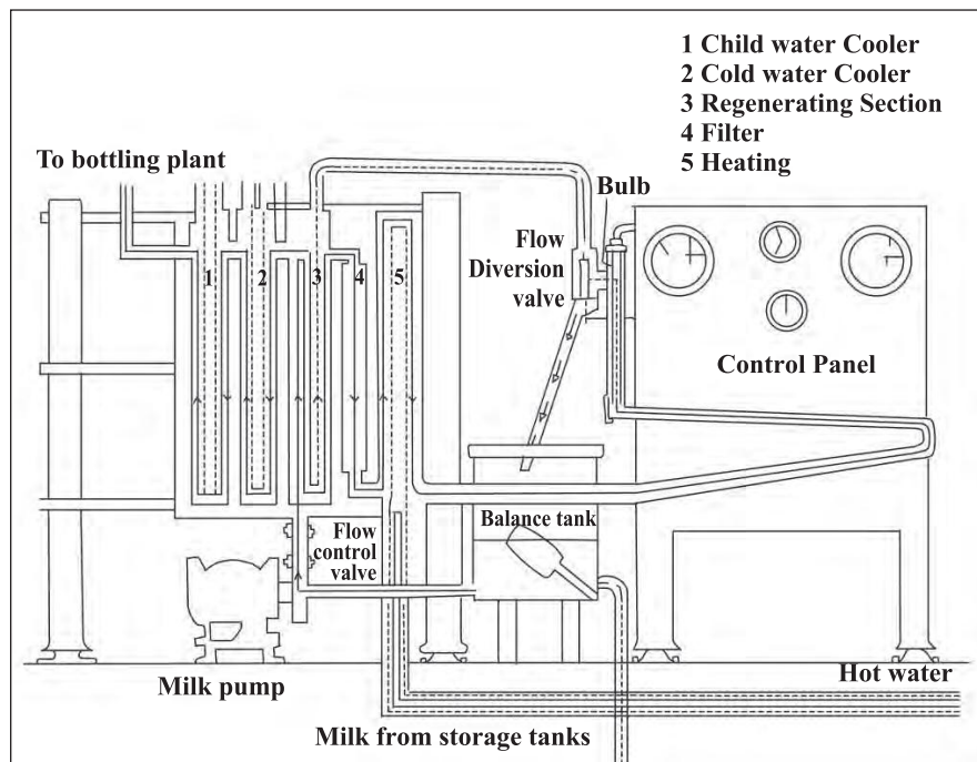
Fig. 9.4 : HTST pasteurizer
