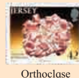
Orthoclase \text{KAlSi}_3\text{O}_8
