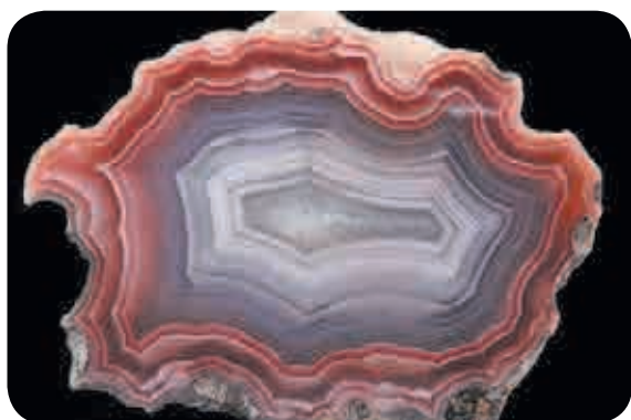
Fig. 5.63 : Agate
