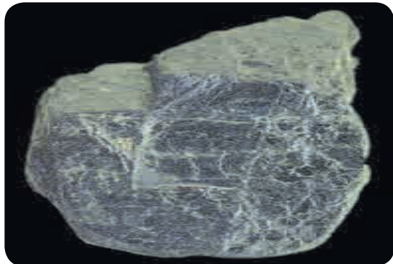
Fig. 5.68 : Hornblende
