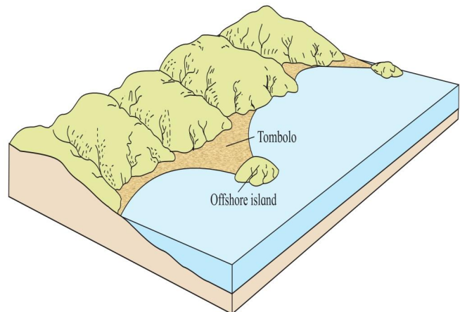
Fig. 3.14 : Tombolo
