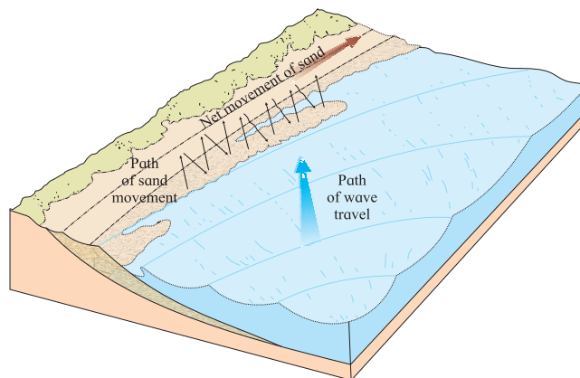
Fig. 3.9 : Longshore drift
