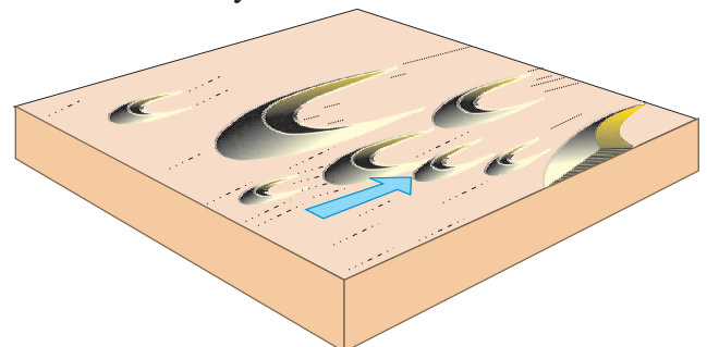
Fig. 3.25 : Barchan dunes
