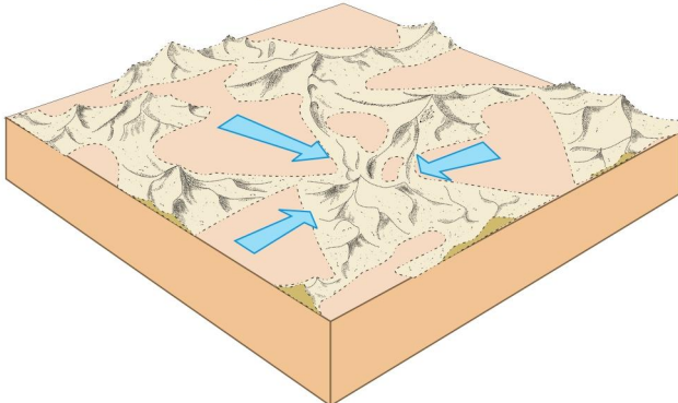
Fig. 3.27 : Star dunes
