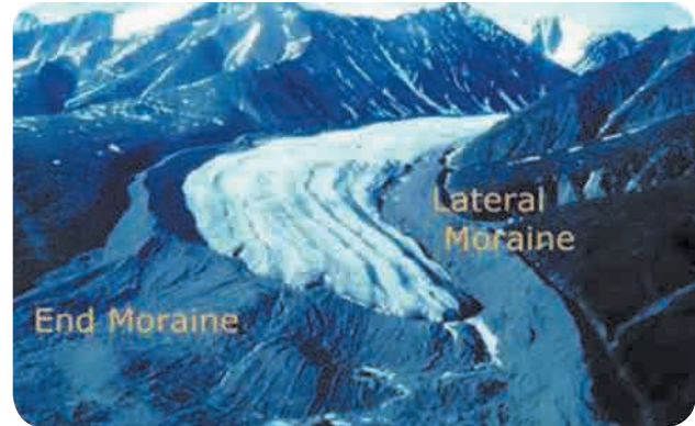
Fig. 3.34 : Glacial moraines
