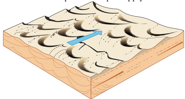
Fig. 3.24 : Transverse dunes
