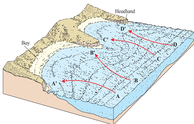
Fig. 3.8 : Wave refraction
