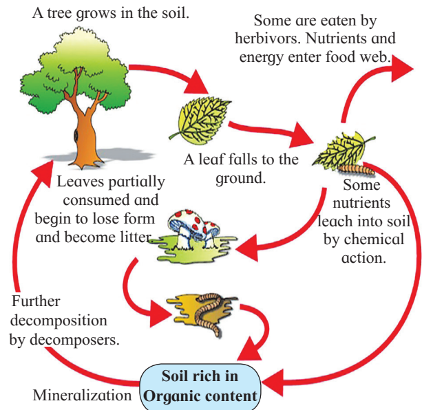
Fig. 14.3 : Decomposition cycle
