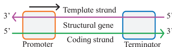
Fig. 4.10 : Transcription unit
